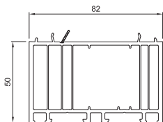
NP8500 Verbreiterung 50 mm
