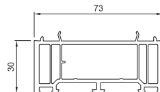
NP1350 Verbreiterung 30 mm
