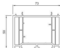
NP1550 Verbreiterung 50 mm
