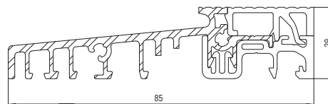
Aluminiumschwelle mit einer thermischen Isolierung
