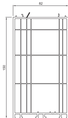
NP8700 Verbreiterung 150 mm
